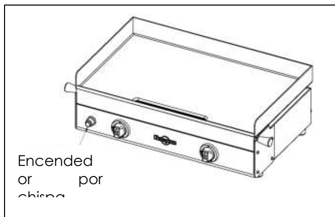
FIGURA 4 – SISTEMA PIEZOELÉCTRICO
