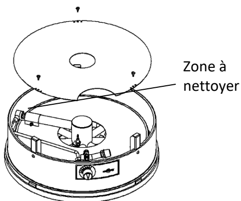
FIGURE 9 – NETTOYAGE ET REGLAGE DU VENTURI
