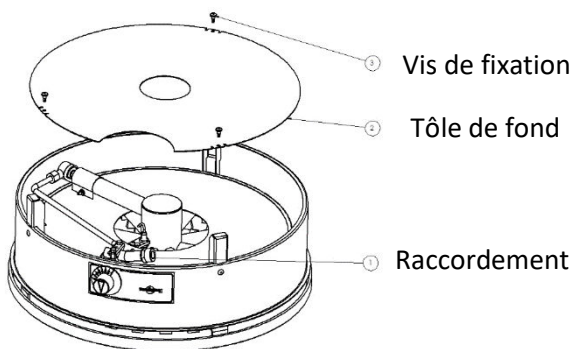
FIGURE 7 – DÉMONTAGE TOLE DE FOND
